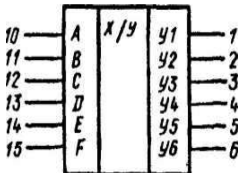
Условное графическое обозначение К155ПР7, КМ155ПР7
