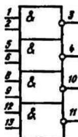
Условное графическое обозначение К561ЛА7, ЭКФ561ЛА7
